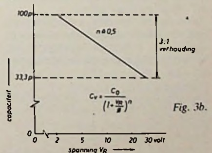
Fig. 3. Conventionele afstemdiode.
